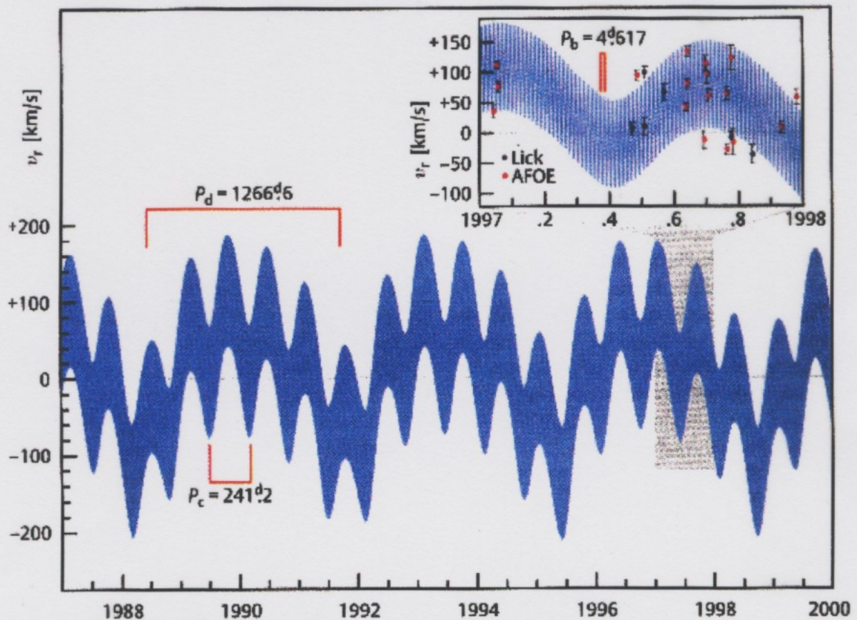
Abb. 9: Die den Messpunkten angepasste Radialgeschwindigkeitskurve von v Andromedae lässt sich als Überlagerung von drei Perioden darstellen – 4.6 Tage (vgl. den vergrößerten Ausschnitt), 241 Tage und 3.47 Jahre. (Butler et al. 1999)
